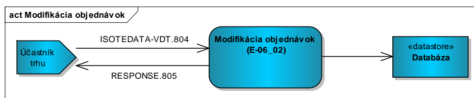
Obrázok 22 Schéma modifikácie objednávky ÚT
