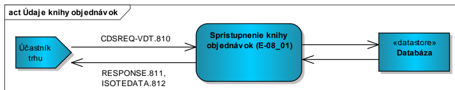
Obrázok 24 Schéma príjmu údajov knihy objednávok
