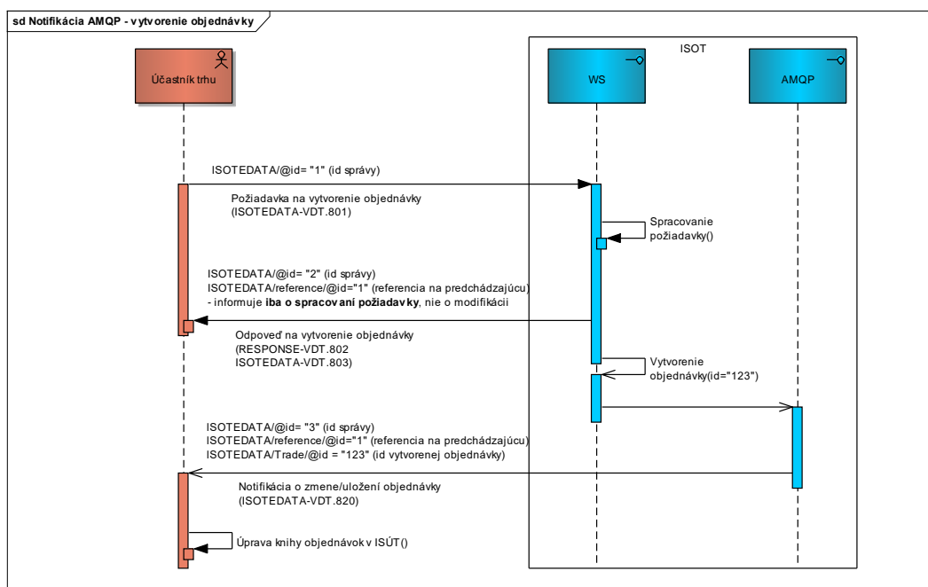
Obrázok 33 Schéma následnosti posielených správ – vytvorenie objednávky (AMQP notifikácia)
