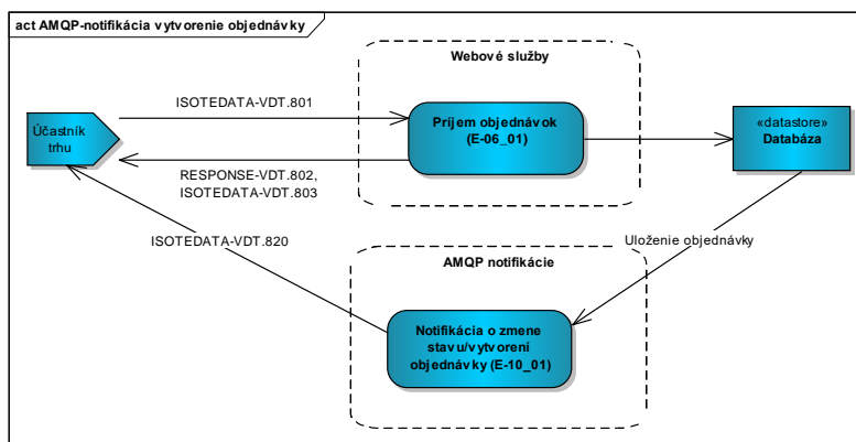
Obrázok 32 Schéma posielených správ – vytvorenie objednávky (AMQP notifikácia)
