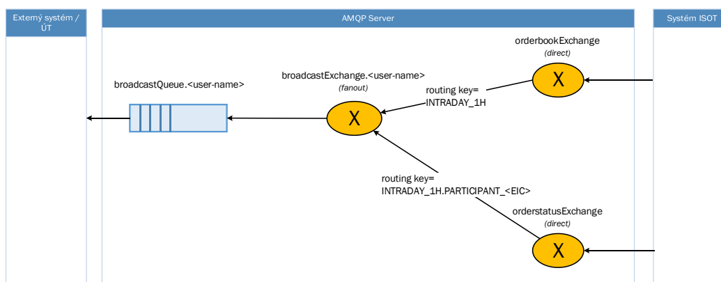
Obrázok 9 Schéma toku notifikačných správ na vnútrodenom trhu
