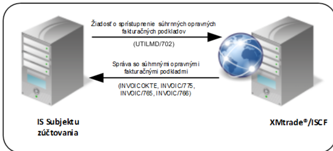
Obrázok 27 Rozhranie pre žiadosť podkladu pre súhrnnú opravnú faktúru
