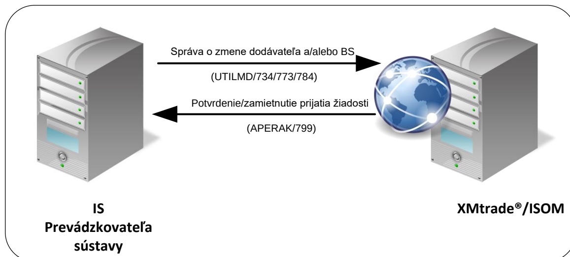
Obrázok 20 Rozhranie pre správu o zmene dodávateľa a/alebo BS
