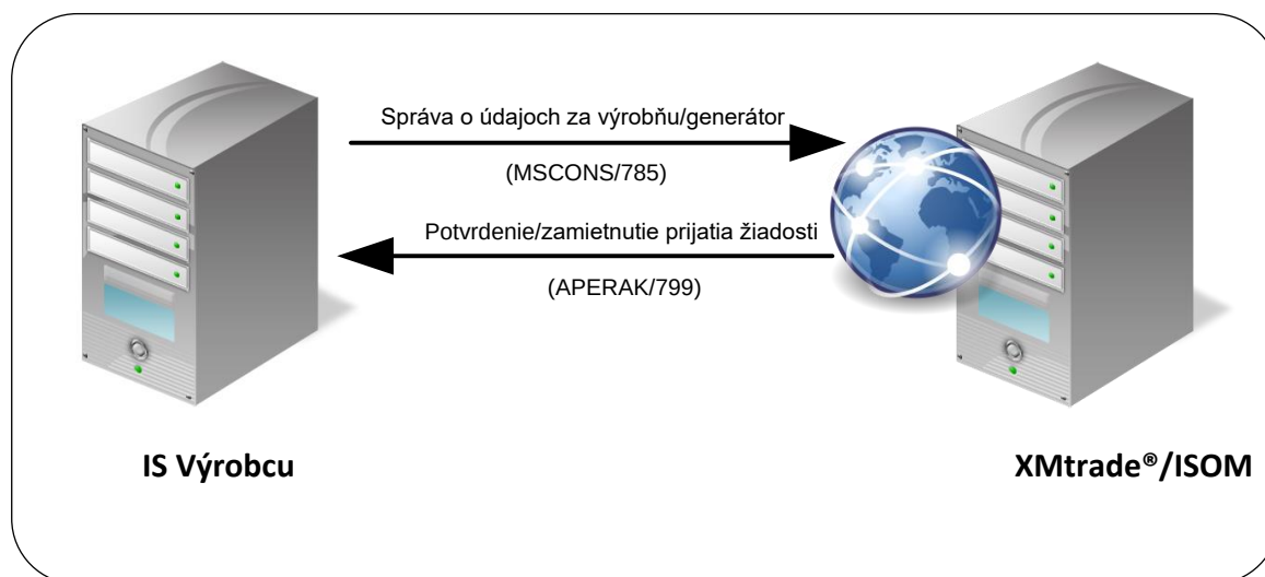
Obrázok 15 Rozhranie pre správu o údajoch za výrobu/generátor
