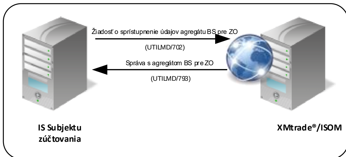
Obrázok 18 Rozhranie pre žiadosť o sprístupnenie údajov agregátu BS pre ZO
