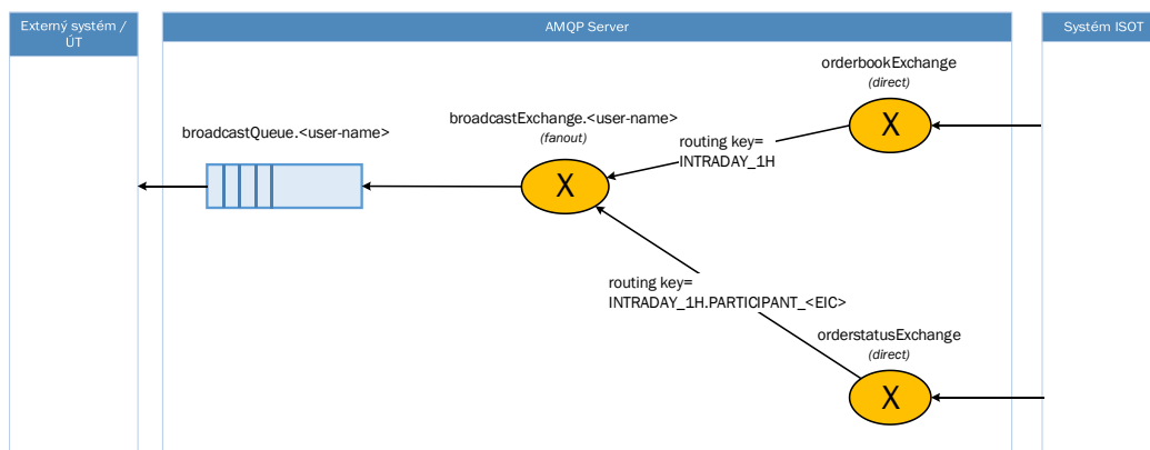
Obrázok 10 Schéma toku notificačných správ na vnútrodenom trhu
