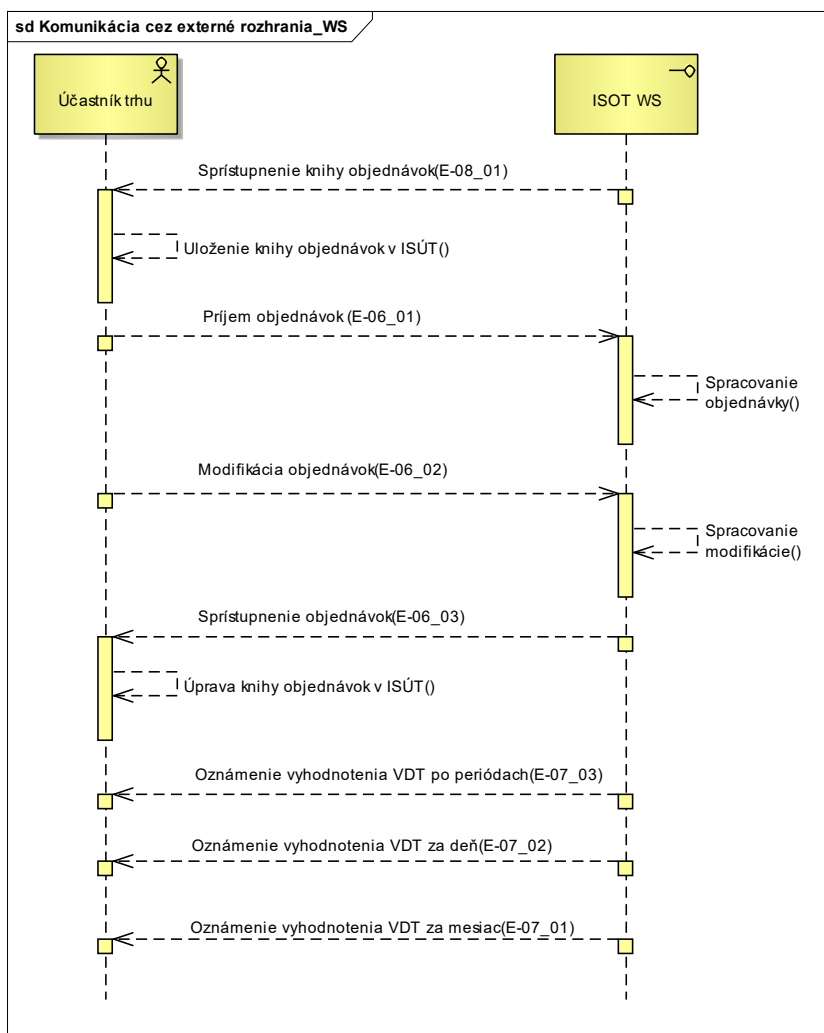
Obrázok 3 Komunikačný scenár webových služieb v režime organizovania domáceho vnútrodeného trhu
